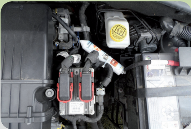
Weber-Isis®-Universal-Aktivator Montage im Motorraum an der Benzinleitung eines Fiat Punto.
